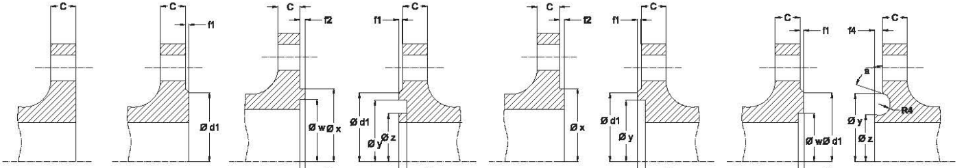
TYP A: Düz yüze TYP B: Conta Yüze TYP C: Uzantı TYP D: Kanallı TYP E: Boru ağızlı TYP F: Girintili TYP G: O-ring ağızlı TYP H: O-ring girintili TYP A: Flat face TYP B: Raised Face TYP C: Tongue TYP D: Groove TYP E: Spigot TYP F: Recess TYP G: O-ring spigot TYP H: O-ring groove
